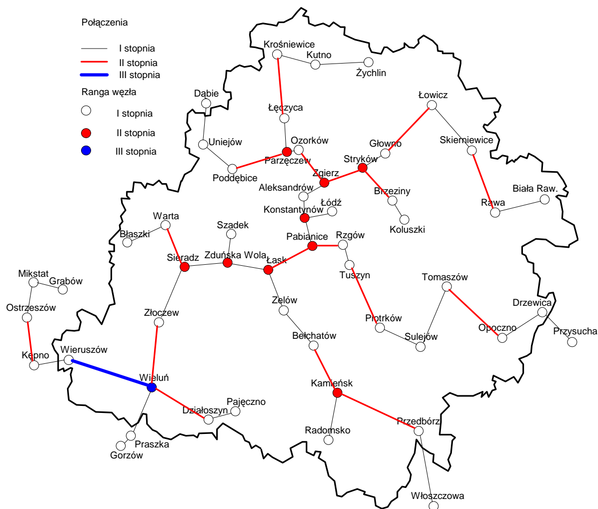
Ryc. 1. Najkrótszy dendryt wrocławski rozpostarty pomiędzy miastami województwa łódzkiego
